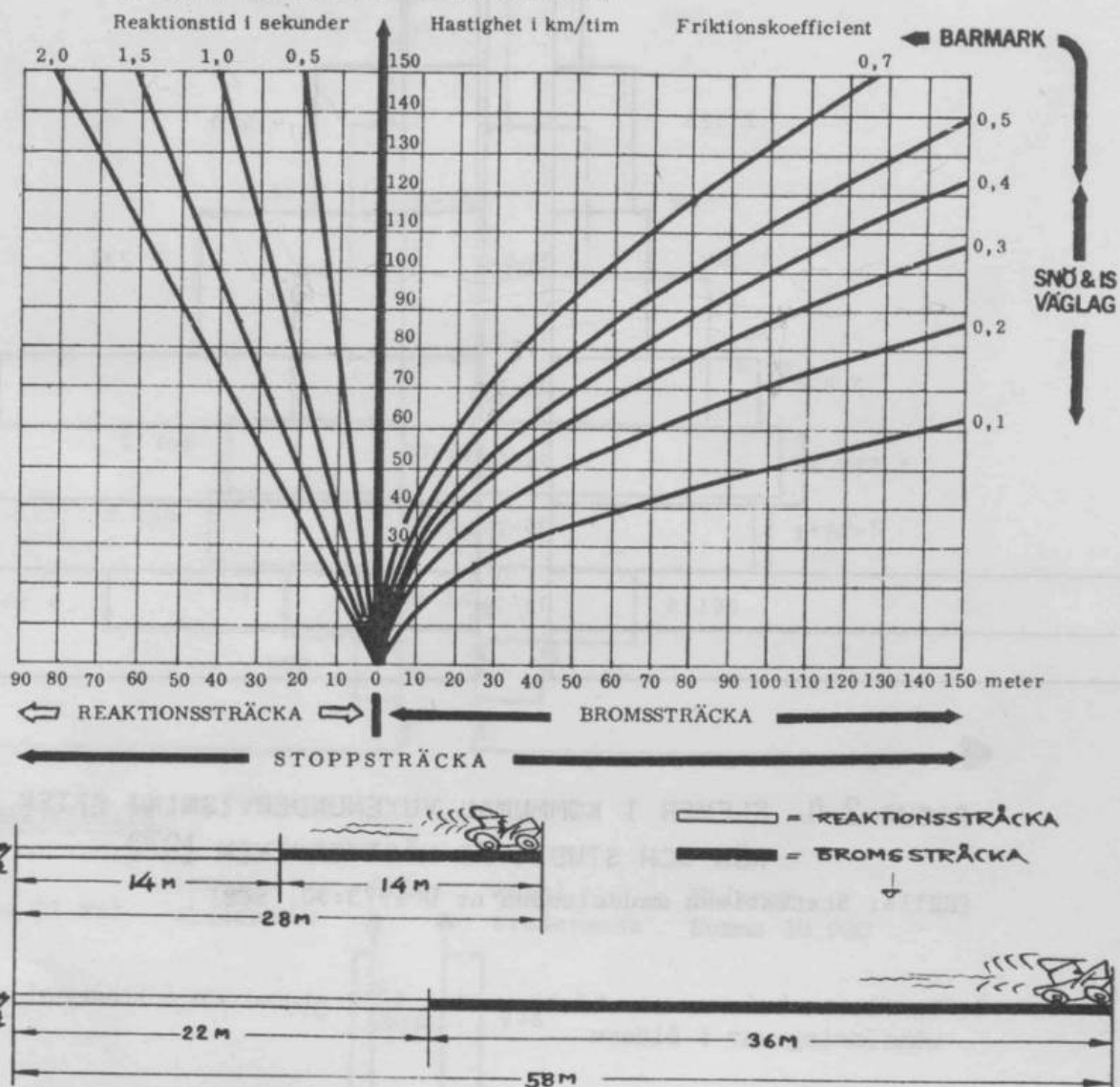
FIGUR 5. STOPPSTRÄCKEDIAGRAM
